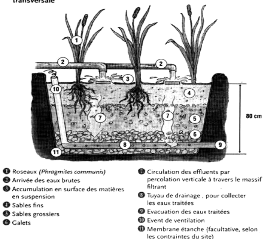
▼ Filtre planté de roseaux à écoulement vertical (FPRV) en coupe transversale
